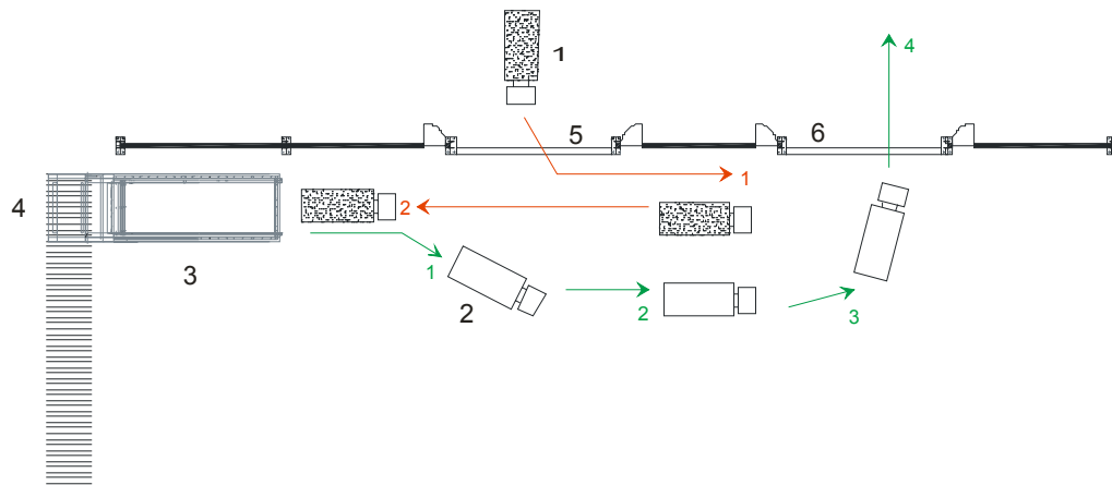
Слика 39 - Шематски приказ маневарских положаја камиона (смећара)
