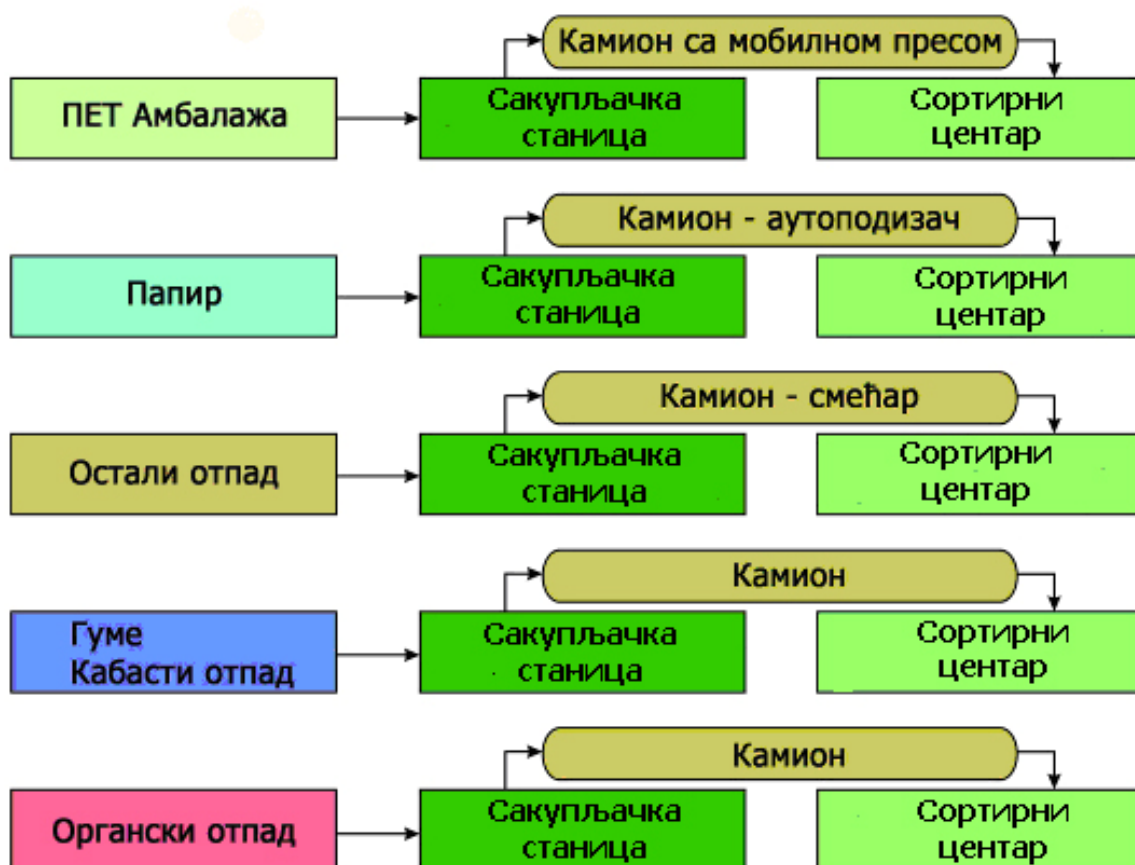
Шема 8 - Шематски приказ сакупљања и транспорта сепарисаног отпада за градско насеље
